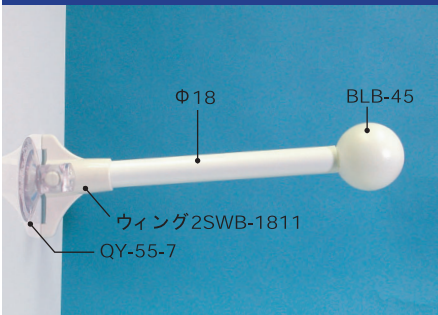
2SWB-QY-18BLB45
